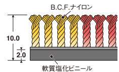
断面形状
