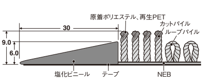
断面形状
