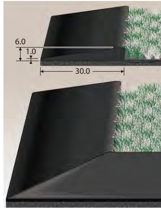
傾斜タイプ 断面イメージ図
